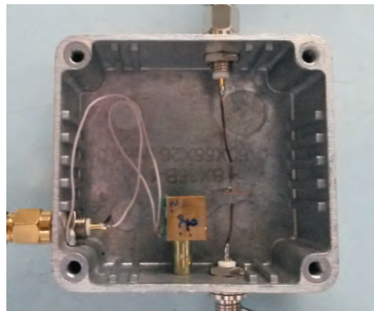
Рис. 1. Схема и фотография макетного образца в экранирующем корпусе
