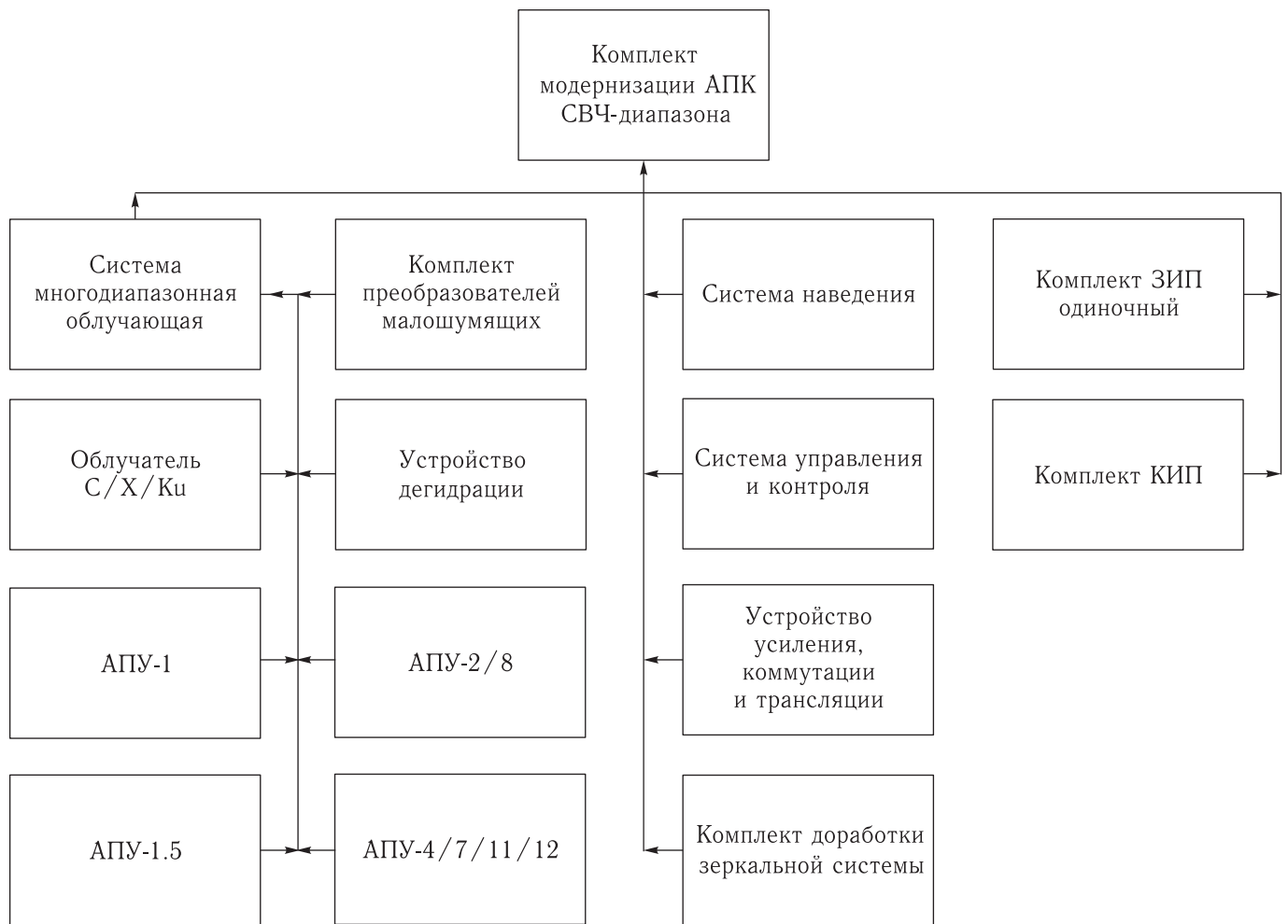
Рисунок. Структурная схема универсальных комплектов модернизации АПК на базе антенных установок ТНА
