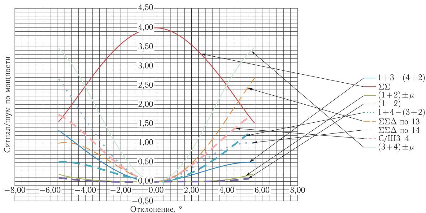
Рис. 15. Отклонение по азимуту. Угол места 75^\circ
