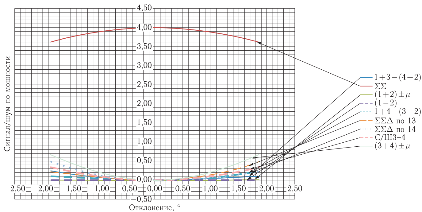
Рис. 16. Отклонение по азимуту. Угол места 85^\circ
