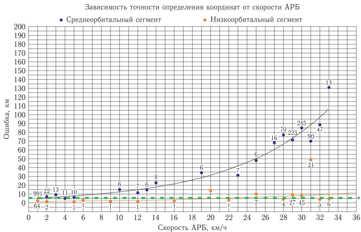
Рис. 2. Результаты определения координат подвижного АРБ с помощью СПОИ-СО ЕС (синие точки), а также с помощью низкоорбитального сегмента КОСПАС-САРСАТ (красные точки)
