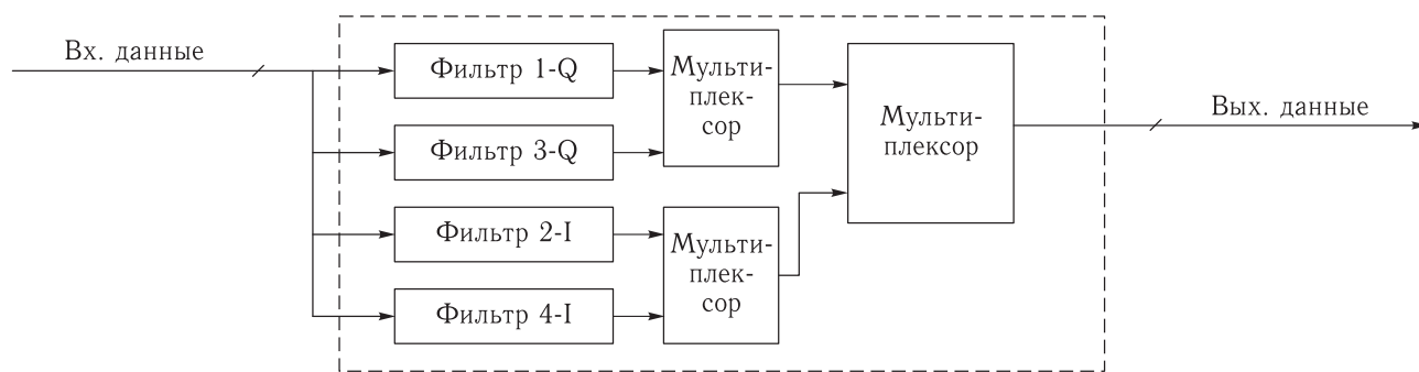
Рис. 6. «Многофазная» (параллельная) структура цифровой фильтрации
