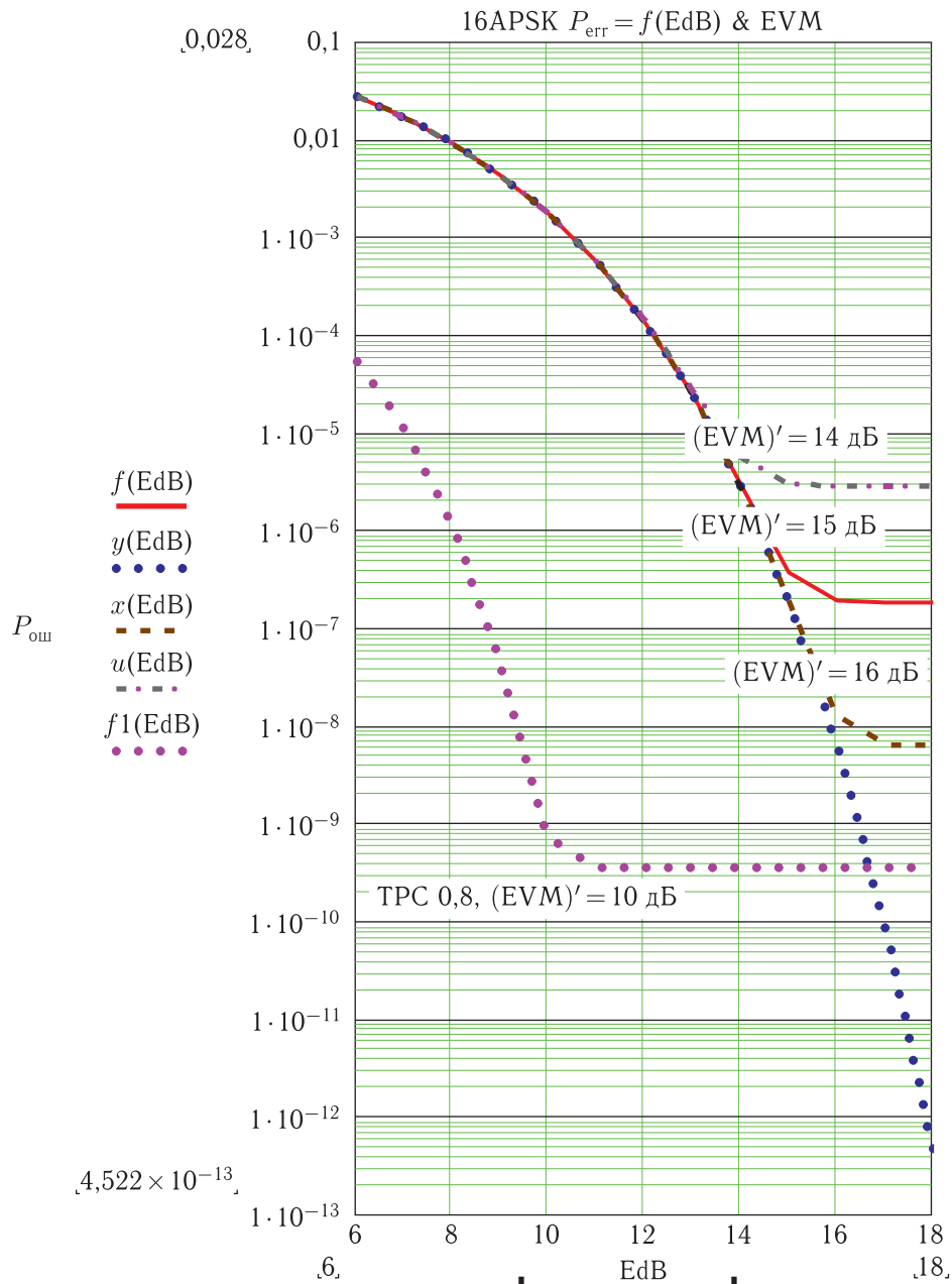
Рис. 7. Кривые зависимости P_{ош} = f(E_{бит}/N_o) при наличии погрешностей формирования сигналов и нелинейности канала
