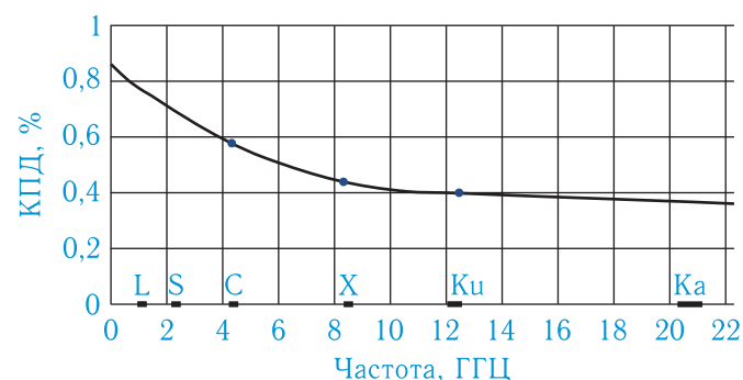
Рис. 4. Прогноз зависимости КПД УМ от частоты
