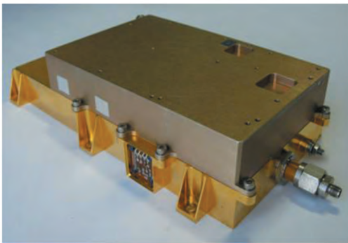
S-диапазон GaN, 80 Вт
